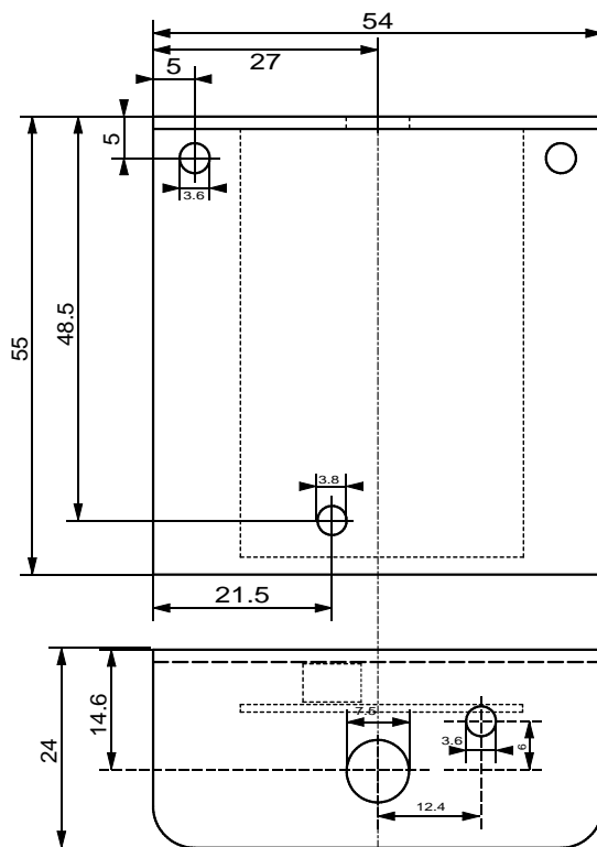
Befestigungswinkel.T3001 Alu 1.5mm 12.06.2024
